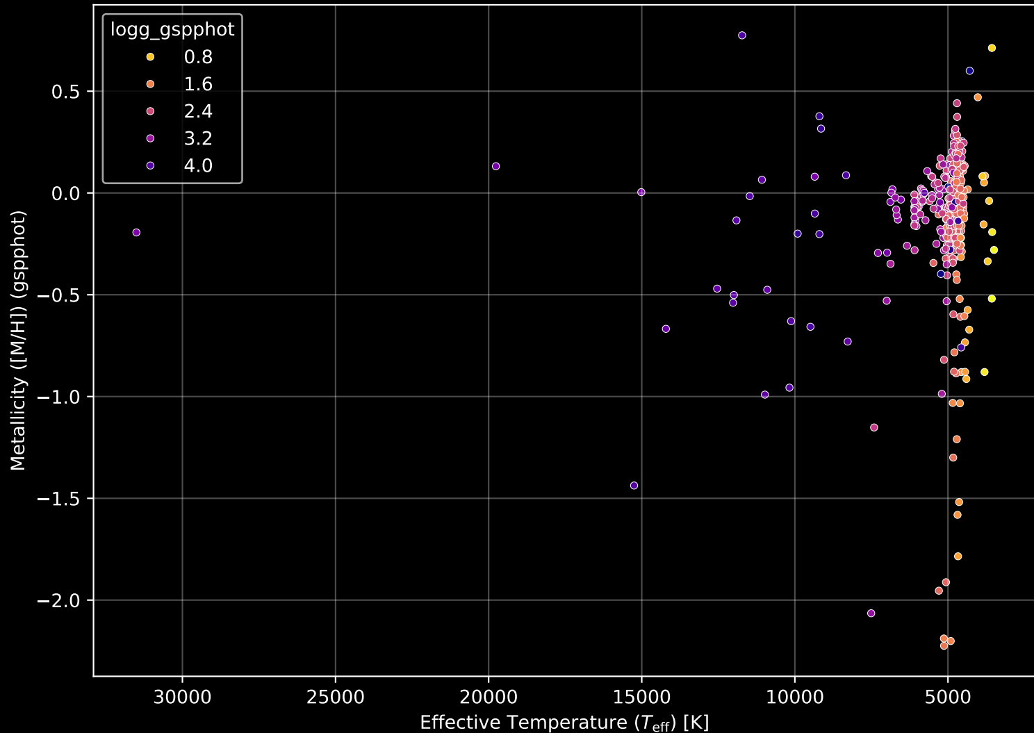
APOGEE DR17 Field: [140+06] Stellar Population Parameters (n= 352)
